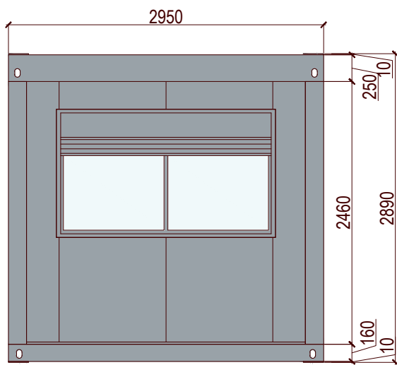
ÉLÉVATION "B"
