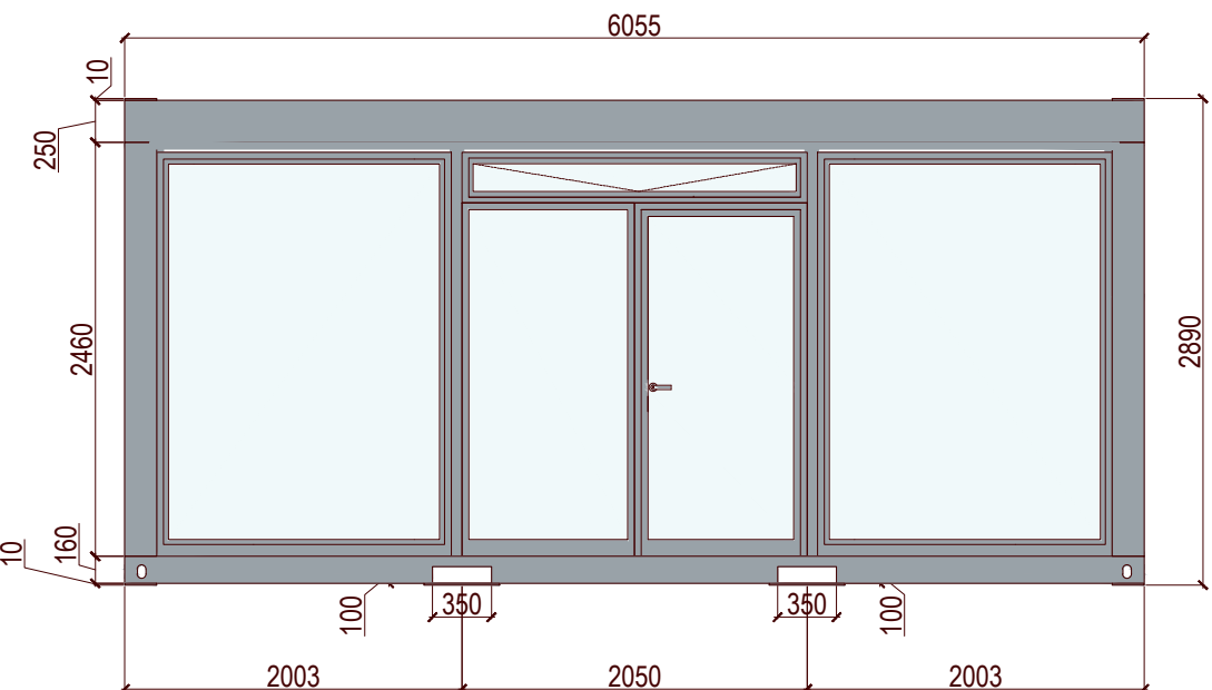
ÉLÉVATION "A"
