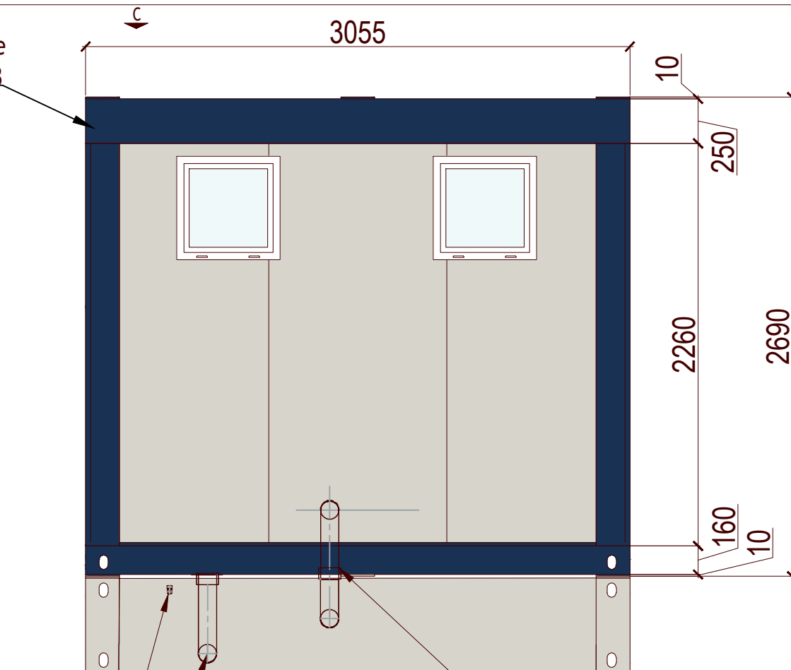
ÉLÉVATION "C"
