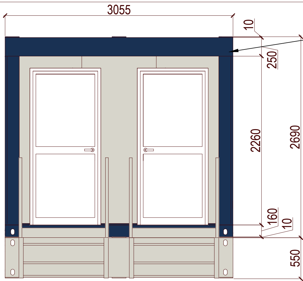
ÉLÉVATION "A"
